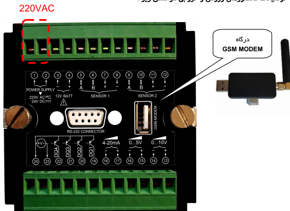
ترتیب سیم بندی و شماره کانکتورها
